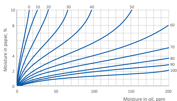
Рисунок 4. Кривые равновесной влажности* (Ооммена)
