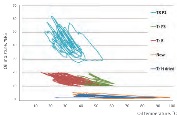
Рисунок 8. Петли гистерезиса относительной насыщенности (%RS) и температуры в трансформаторе при различных уровнях влажности*
